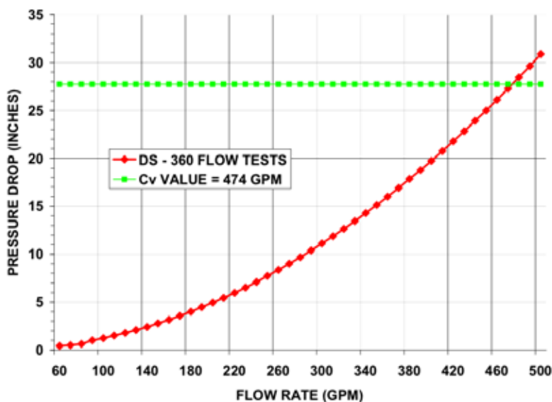
DS - 360 FLOW TESTS / Cv VALUE
